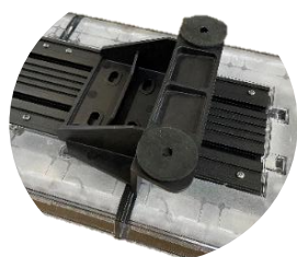
Fixation pattes réglables avec 4 silent-blocs
