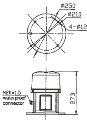
Installation( mm)
