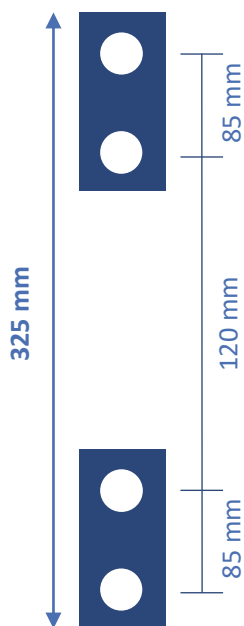
Schéma de perçage
